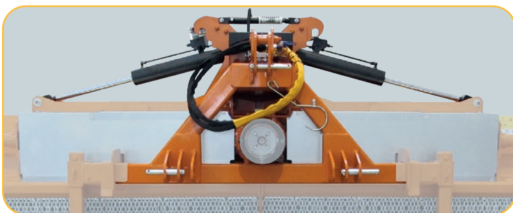
- 3-pkt. stały układ zawieszenia z hakami hydraulicznymi do rozkładania/składania, Kat. 2-3 - Fixed 3-point linkage, Cat. II-III and hydraulic hooks for open/close
