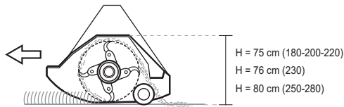
- Przednie łańcuchy ochronne - Front chains protectors
