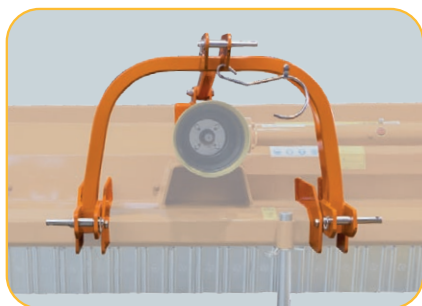
- 3-pkt układ zawieszenia, stały, Kat. 2 - Fixed 3-point linkage, Cat. II
