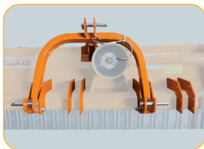
- 3-pkt układ zawieszenia, stały, Kat. 2. (regulowany w dwóch pozycjach tylko dla 230) - Fixed 3-point linkage, Cat. II (adjustable in two positions only for 230)
