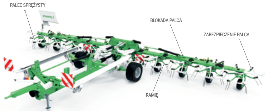
PALEC SPRĘŻYSTY
