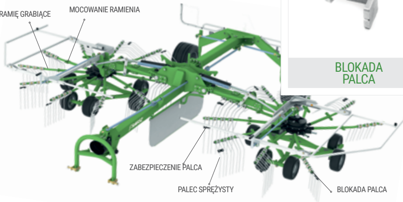
MOCOWANIE RAMIENIA
