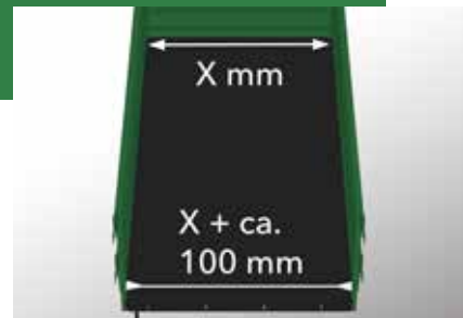
Stożkowa podłoga z blachy stalowej gwarantuje łatwe zsuwanie się ładunku
